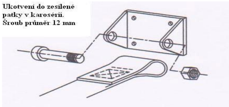
Obr.4 - Příklad uchycení ramenního pásu do karosérie
